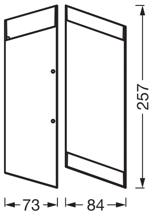
ENDURA STY COPEN UPD W 10W IP54 DG
