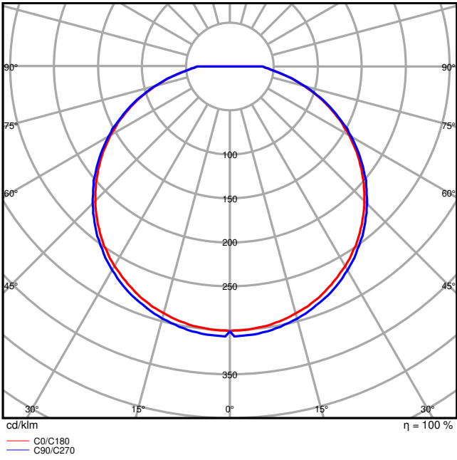
SF SLIM SQ 200 P 19W 840 IP65 WT
