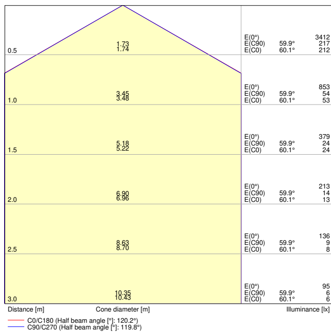
SF SLIM RD S 260 P 26W 840 IP65 WT
